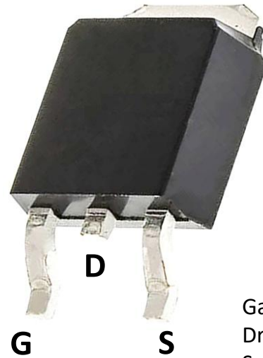
GR-65J240JA (TO-252)
